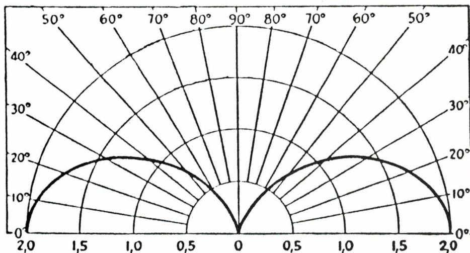
Fig. 5 Vertikale antenne
