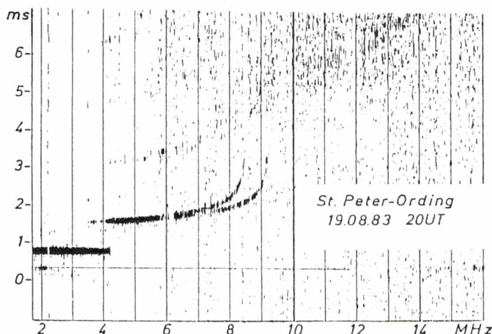
Fig. 2 Reflectie diagram
