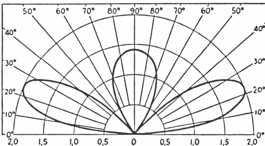
Fig. 4b Draadantenne op 5/8 golflengte boven de grond
